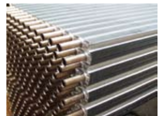
PLATEFIN
